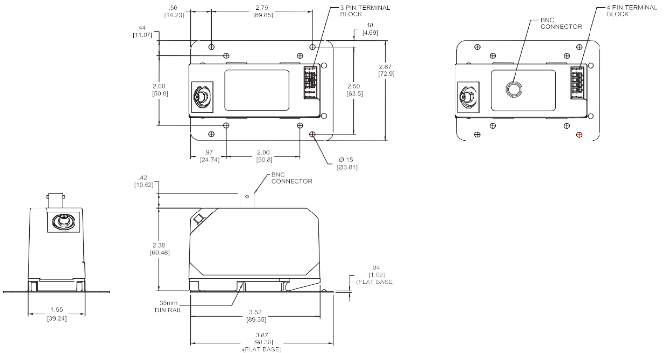
図2. 『MX2034 デジタル近接トランスミッタ』(『取付金具 9647』も併記)
