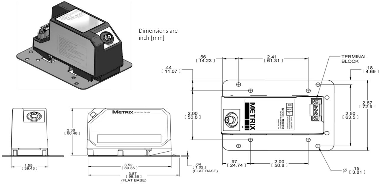
図1. 『MX2033 3線式デジタル近接ドライバ』(『取付金具 9647』も併記)
