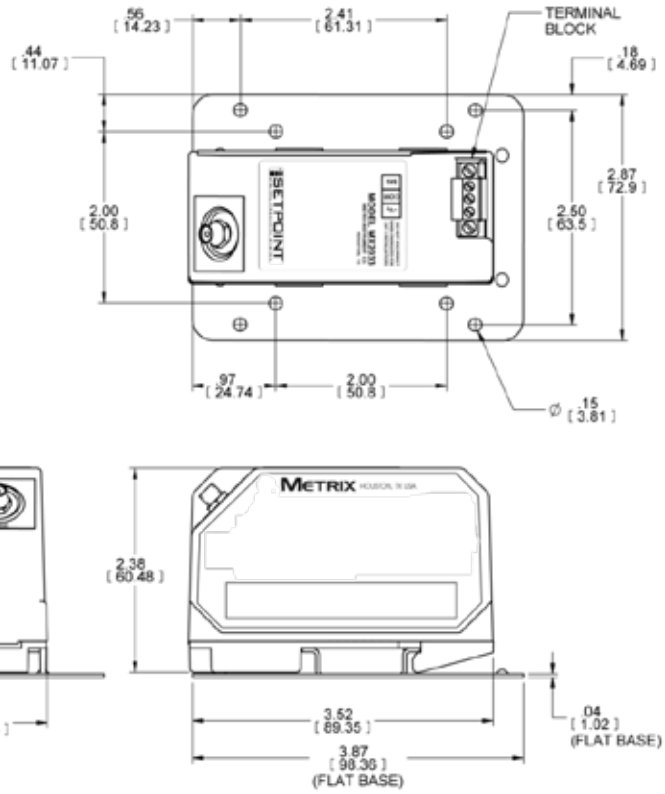
图 1: MX2033 3-线制数字趋近式前置器尺寸 单位: 英寸[MM] 说明: 图示可选的4孔底板安装支架。标准的是35MM DIN导轨安装。
