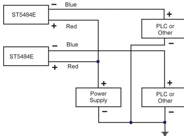
図2. 『ST5484E』 (複数信号配線)
