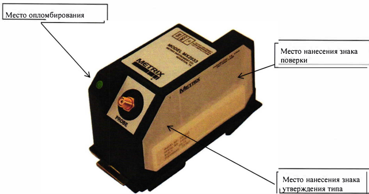
Рисунок 2 – Внешний вид трансмиттеров/драйверов MX2033 и MX2034
