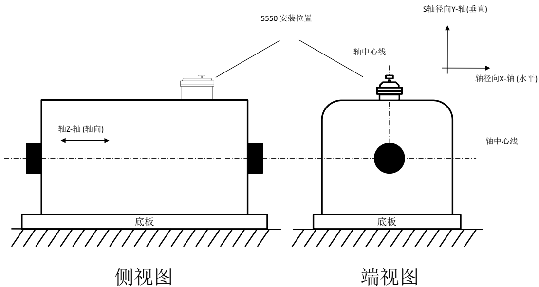
图G: 水平机器显示垂直5550安装方向 (不推荐)
