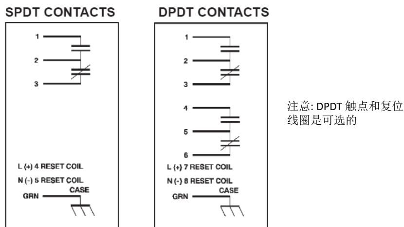
图L: 5550接线
